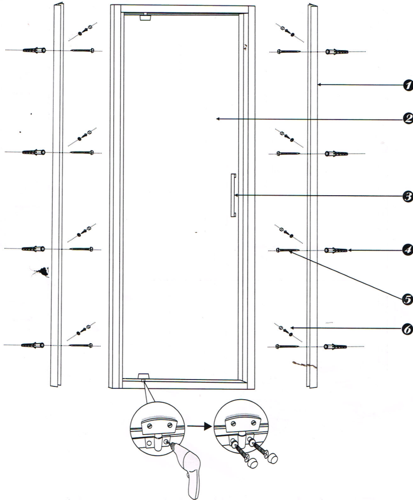
Pivot Door
